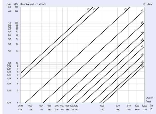
DN 25 - Innen-/Innengewinde
