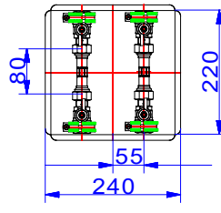
Wassergarge W2-Typ A
