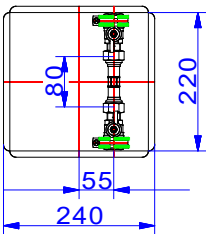
Wassergarge W1-Typ A
