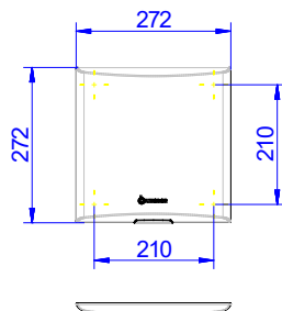
Abdeckblende LIM Premium
