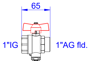
Fühleranschlussstück 5mm M10x1 55-005096
