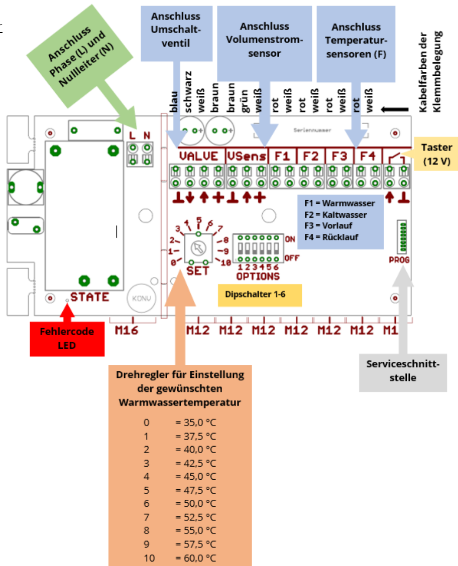
Klemmbelegung Regler
