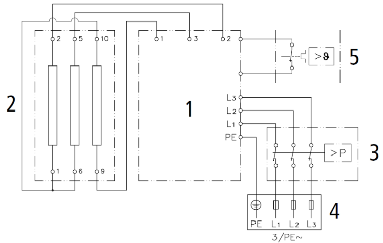
Schaltplan:
